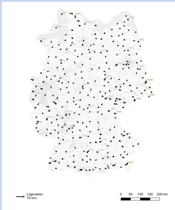
Abb. 1+2: Vergleich der beiden Netz-B-Berechnungsvarianten (Restklaffungen nach der zwangsfreien Auffelderung der Variante AMK auf die Variante RFK, LGLN-Auswertung)
